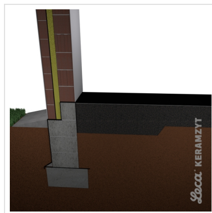
4. Izolacja przeciwwilgociowa (np. 2 x folia)
