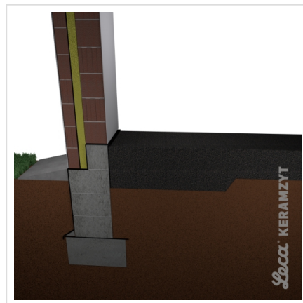
2. Warstwa Leca® KERAMZYTU impregnowanego
