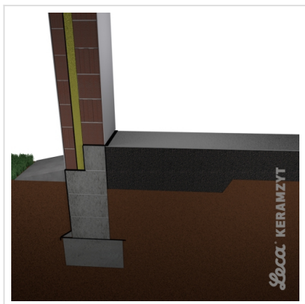
3. Szpryc cementowy wzmacniający górną powierzchnię keramzytu
