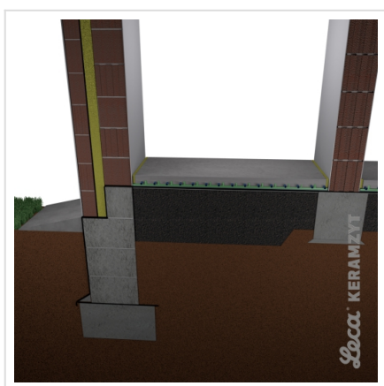
9. Jastrych cementowy zbrojony
