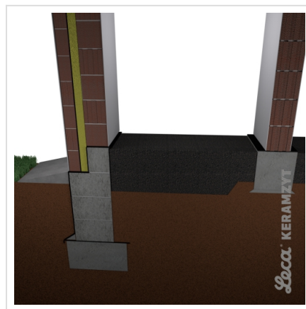
4. Warstwa Leca® KERAMZYTU impregnowanego
