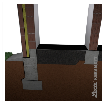
6. Izolacja przeciwwilgociowa (np. 2 x folia)
