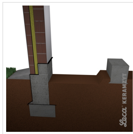
2. Podkład i fundament pod ściankę
