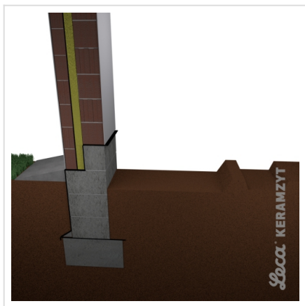
1. Wykop i wyrównanie podłoża
