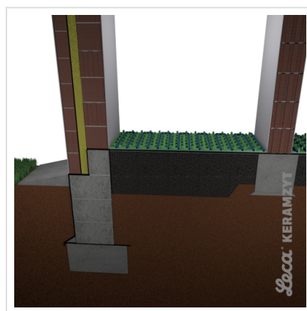
8. Rurki ogrzewania na macie kształtującej ich trasę
