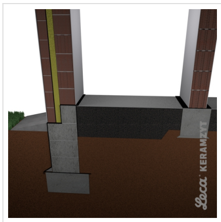
5. Szpryc cementowy wzmacniający górną powierzchnię keramzytu
