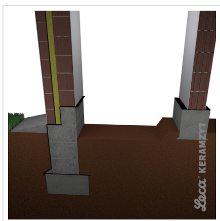
3. Izolacja pozioma i ścianka działowa
