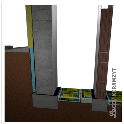
5. Przecięcie górnej folii worków i zasypanie szczelin
