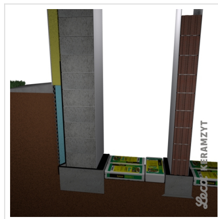
4. Ułożenie worków z Leca® KERAMZYTEM izolacyjnym L
