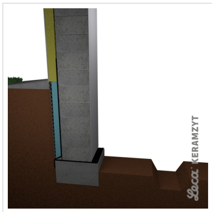
1. Wyrównanie podłoża w piwnicy i wykop pod dodatkowy fundament
