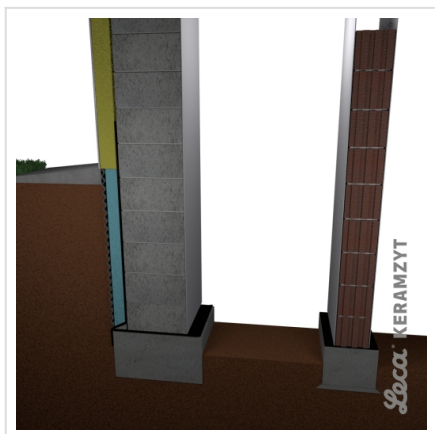
3. Izolacja dodatkowa na fundamencie i ścianie z tynkiem
