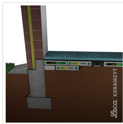
8. Dodatkowa izolacja płytowa (np. styropian EPS, XPS)
