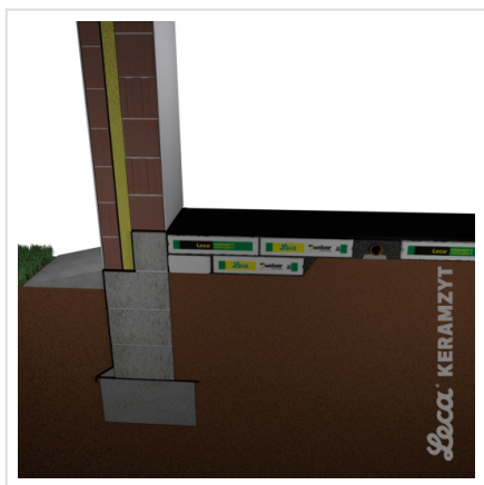
7. Izolacja przeciwwilgociowa (np. 2 x folia)
