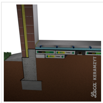
11. Jastrych cementowy zbrojony
