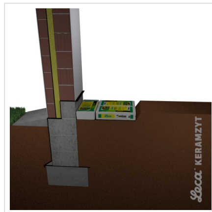
2. Ułożenie worków z Leca® KERAMZYTEM izolacyjnym L pierwsza warstwa
