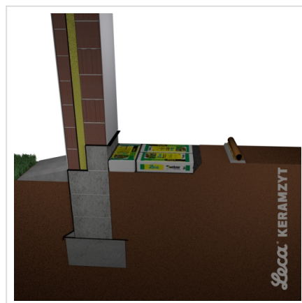
4. Podsypka i rura instalacyjna
