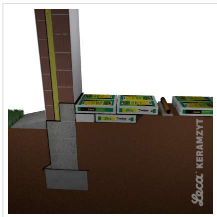
5. Ułożenie worków z Leca® KERAMZYTEM izolacyjnym L druga warstwa
