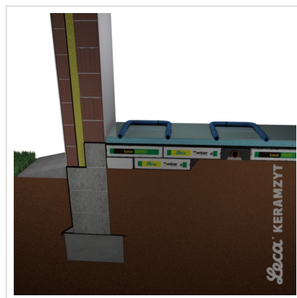
10. Rurki ogrzewania montowane na izolacji płytowej
