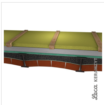
9. Wełna mineralna pomiędzy legarami 1 cm poniżej wierzchu legara
