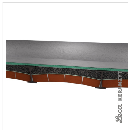
6. Jastrych cementowy zbrojony min. 5 cm
