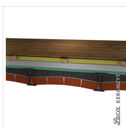
10. Podłoga z desek
