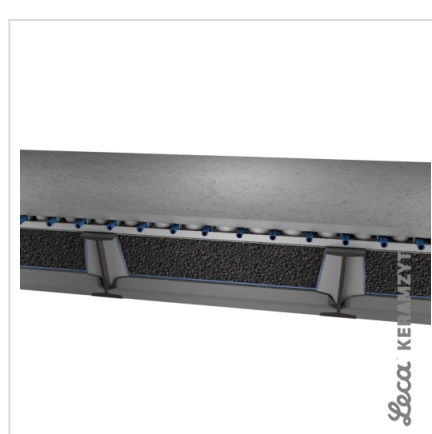
6. Płyty suchego jastrychu
