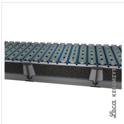
5. Rurki ogrzewania na folii metalizowanej i specjalnej macie izol. kształtującej ich trasę
