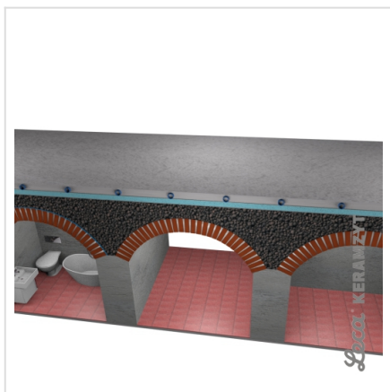
7. Jastrych cementowy zbrojony
