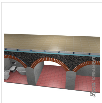
9. Posadzka
