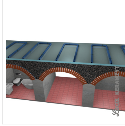
6. Rurki ogrzewania montowane na izolacji płytowej
