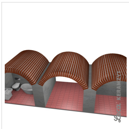
1. Sklepienie łukowe
