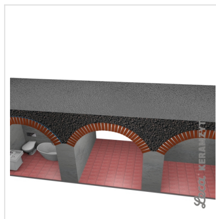
4. Szpryc cementowy
