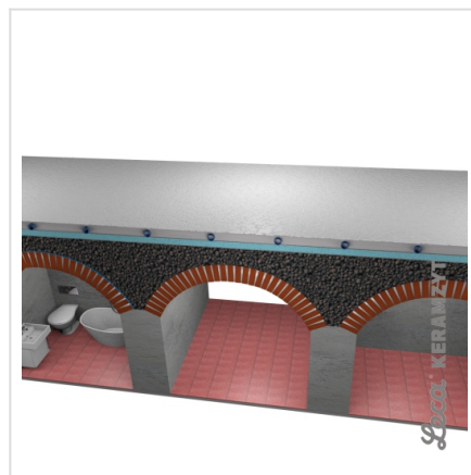
8. Hydroizolacja
