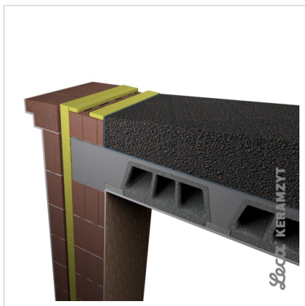
3. Izolacja z Leca® KERAMZYTU izolacyjnego L
