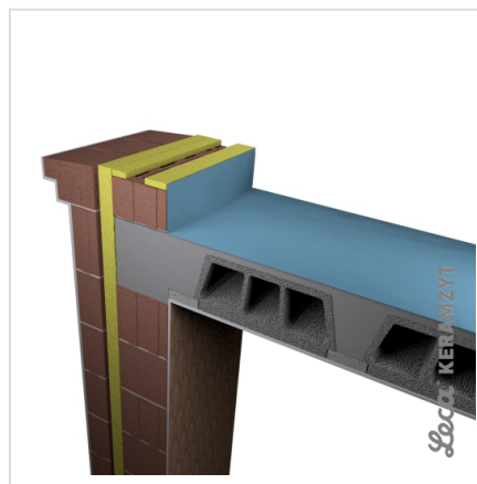
2. Paroizolacja na stropie
