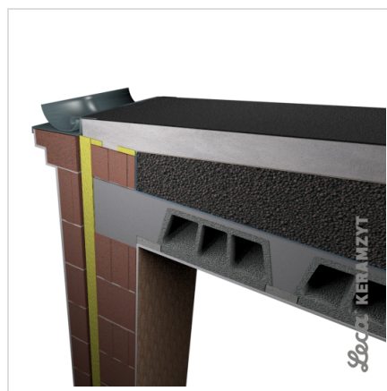
6. Bitumiczne pokrycie dachu
