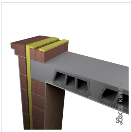
1. Strop ostatniej kondygnacji
