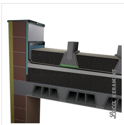
9. Drenaż z Leca® KERAMZYTU budowlanego L w geowłókninie
