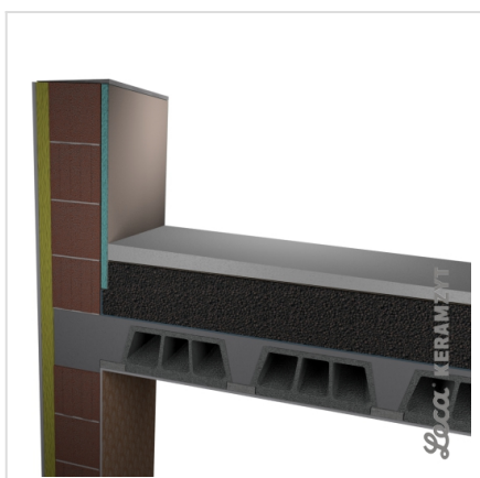
5. Jastrych kształtujący spad
