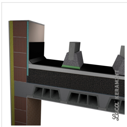
7. Obrzeża na ławach z lekkiego betonu z przepustami
