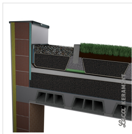
10. Nawierzchnie zielonego dachu
