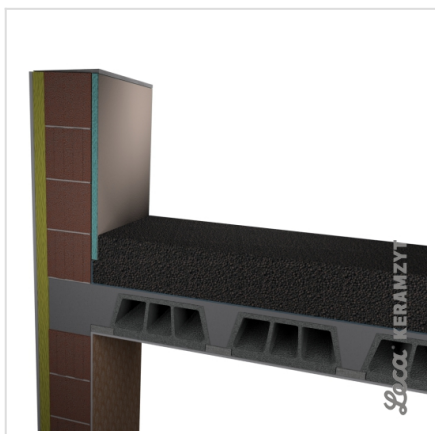
3. Izolacja termiczna z Leca® KERAMZYTU izolacyjnego L
