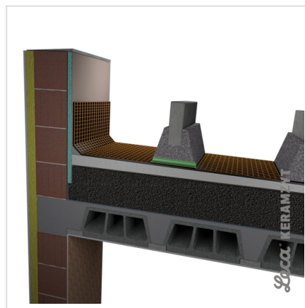
8. Folia lub siatka przeciw przerastaniu korzeni
