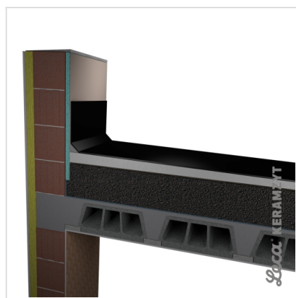
6. Hydroizolacja
