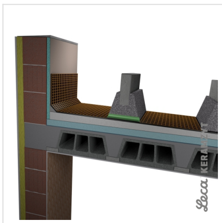
7. Folia lub siatka przeciw przerastaniu korzeni
