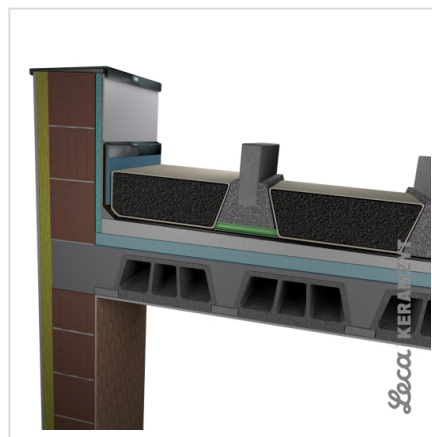
8. Drenaż z Leca® KERAMZYTU budowlanego L w geowłókninie
