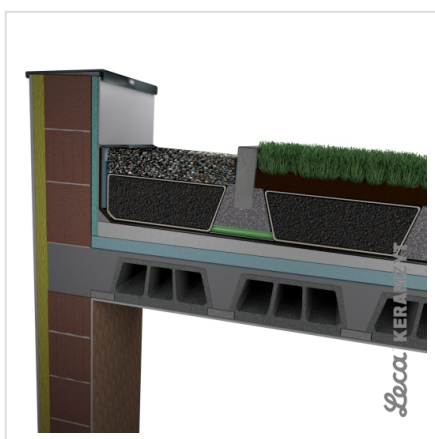
9. Nawierzchnie zielonego dachu
