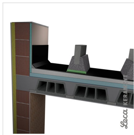
6. Obrzeża na ławach z lekkiego betonu z przepustami
