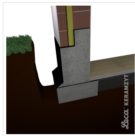
2. Izolacja przeciwwilgociowa ścian
