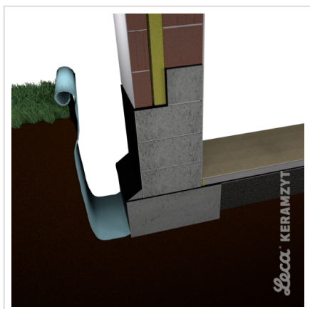
3. Geowłóknina separacyjna na dnie i ścianach wykopu z zapasem
