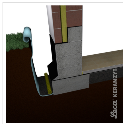
4. Rura drenarska na warstwie keramzytu lub piasku
