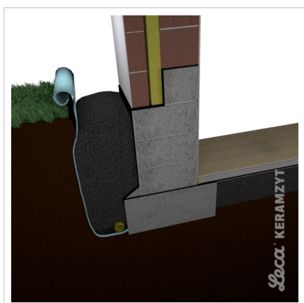
5. Wypełnienie wykopu Leca® KERAMZYTEM budowlanym L
