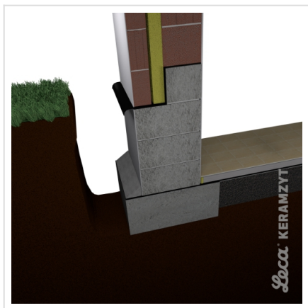
1. Wykop obwodowy wzdłuż ścian piwnicznych
