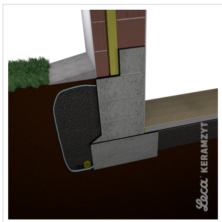
7. Wyrównanie gruntu i ew. ułożenie opaski betonowej
