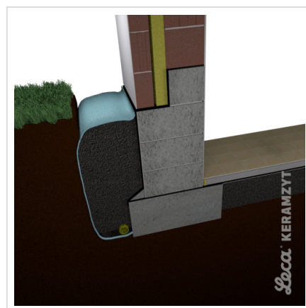
6. Przykrycie wypełnienia geowłókniną
