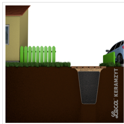
6. Przepuszczalna nawierzchnia chodnika
