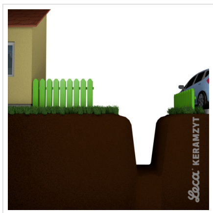
1. Wykop wzdłuż drogi
