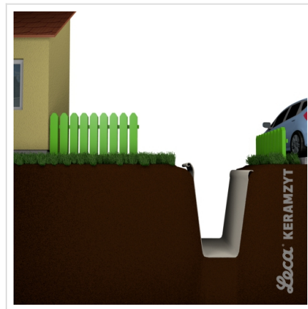
2. Geowłóknina separacyjna na dnie i ścianach wykopu z zapasem
