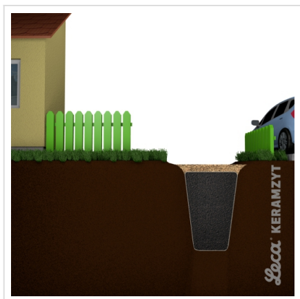
5. Podsypka piaskowo żwirowa
