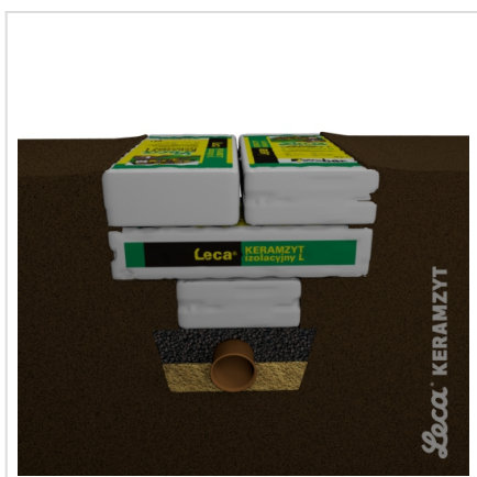
5. Przykrycie rur kolejnymi warstwami worków
