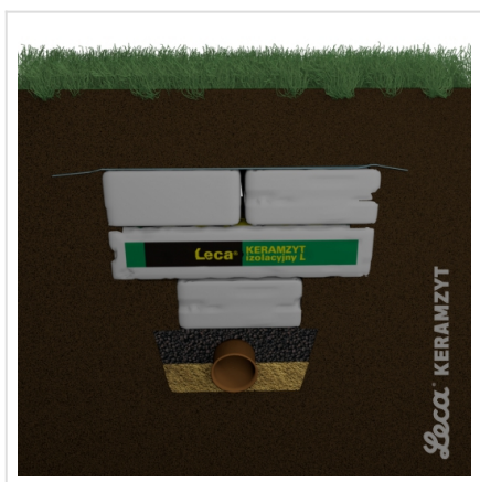
7. Wyrównanie terenu i ew. podbudowa oraz nawierzchnia
