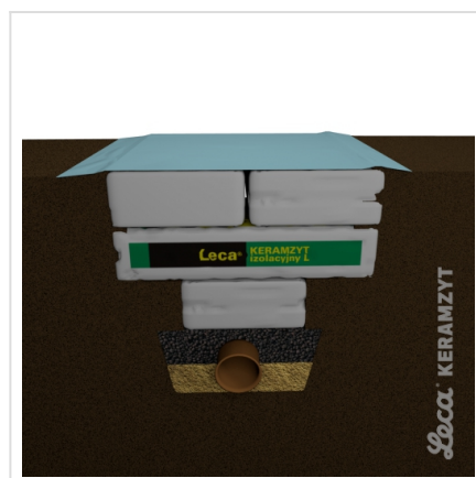
6. Folia przykrywająca izolację
