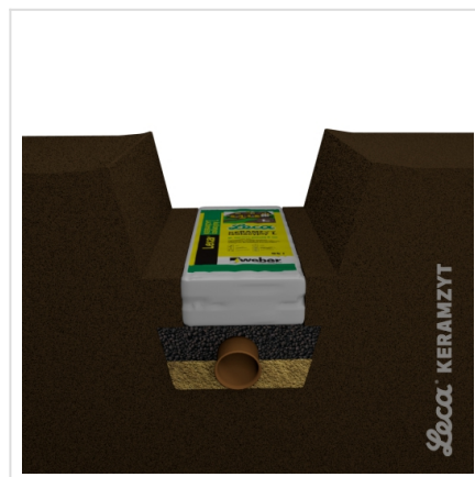
4. Przykrycie rur warstwą Leca® KERAMZYTU izolacyjnego L w workach
