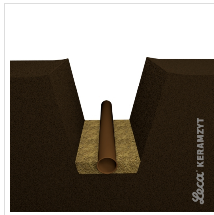
2. Podsypka piaskowa i rura instalacyjna
