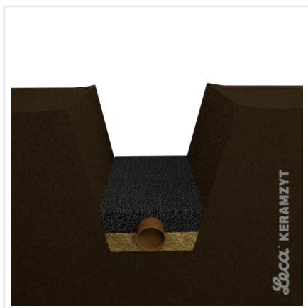
3. Obsypanie rury Leca® KERAMZYTEM izolacyjnym L
