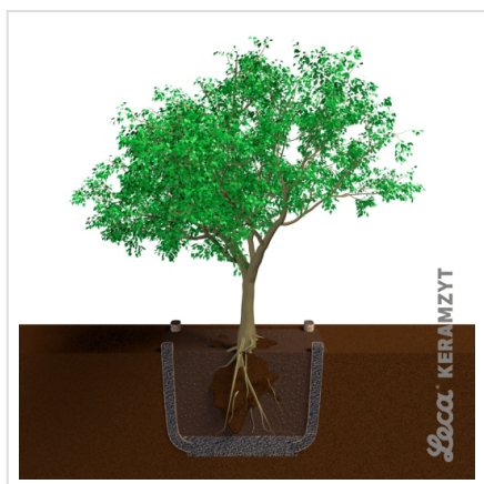
5. Obsypanie korzeni ziemią urodzajną z dodatkiem spulchniającego Leca® KERAMZYTU ogrodniczego M lub L
