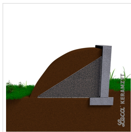
6. Obsypanie górki ziemią urodzajną
