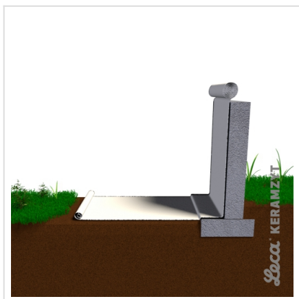
3. Ułożenie agrowłókniny separacyjnej z zapasem
