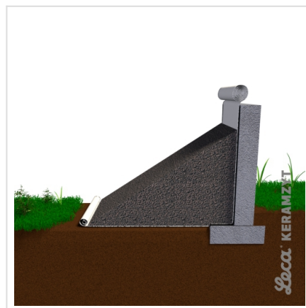
4. Usypanie górki z Leca® KERAMZYTU ogrodniczego L
