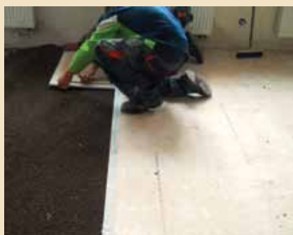
Układanie płyt na Leca® KERAMZYCIE podsypkowym.
